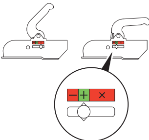
fig. 5: Indicateur de l'usure
