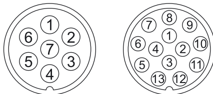
Abb. 1: Steckeranfertigungen
