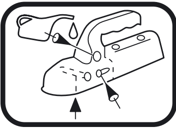
Abb. 3: Aufkleber Schmierpunkte der Kupplung
