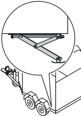
Abb. 12: Abstellstütze
